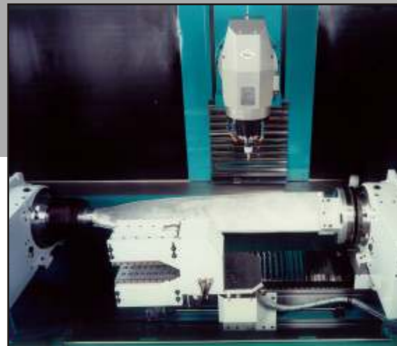
Speciale per industria aerospaziale Special configuration for aerospace Sonderausführung für Raumfahrtindustrie Configuration spéciale pour l'industrie aéronautique
