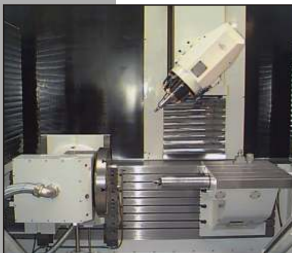
Divisore girevole e basculante per lavorazioni a 4 / 5 assi. CN rotary and tilting table for 4 / 5 axes machining. NC Teilgerät, schwenkbar, zur 4 / 5 Achsen-Bearbeitungen Diviseur tournant et basculant pour usinage à 4 / 5 axes.
