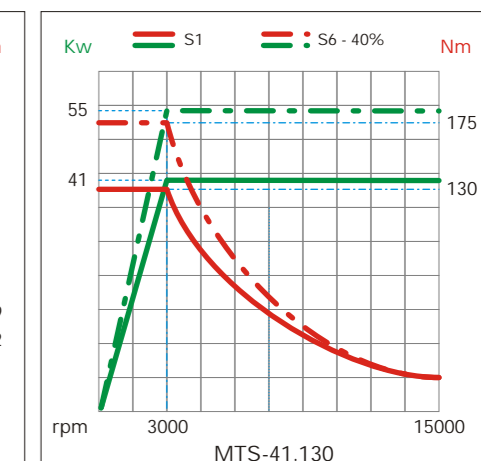
Motore AC sincrono • Synchronous-motor Synchron-Motor • Moteur synchrone
