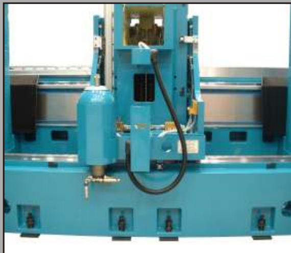
Movimento XY con motore lineare XY travels with linear motor XY Fräsweg mit Linear-Motoren Course XY avec moteurs linéaires
