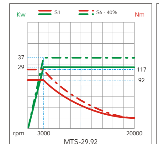
Motore AC sincrono • Synchronous-motor Synchron-Motor • Moteur synchrone
